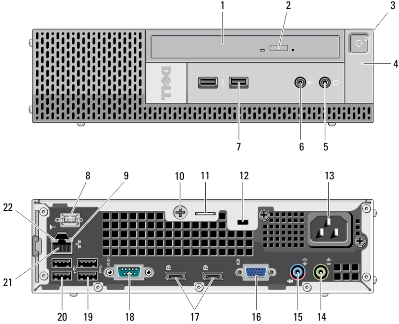
Rakam 6. Ultra Small Form Factor Önden ve Arkadan Görünüm
