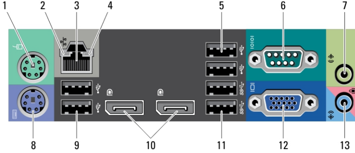
Rakam 3. Mini Tower Ve Masaüstü Arka Panel Görünümü
